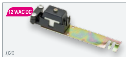
NIEDERVOLT-DISTANZBÜGEL UNIVERSAL
